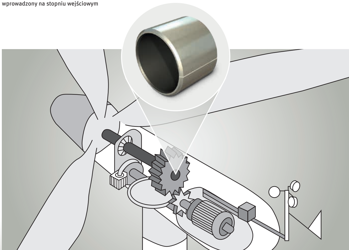
Łożyska ślizgowe PERMAGLIDE® P10 stosuje się jako łożyska prowadzące wałów rotorów w przekładniach elektrowni wiatrowych
