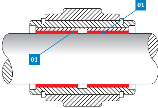
01 KS Permaglide® kaymalı yatak burcu Yapı türü PAP ... P200
