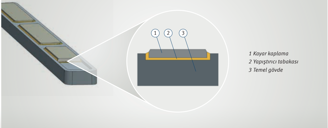
Yapıştırılmış kayar çubuk
