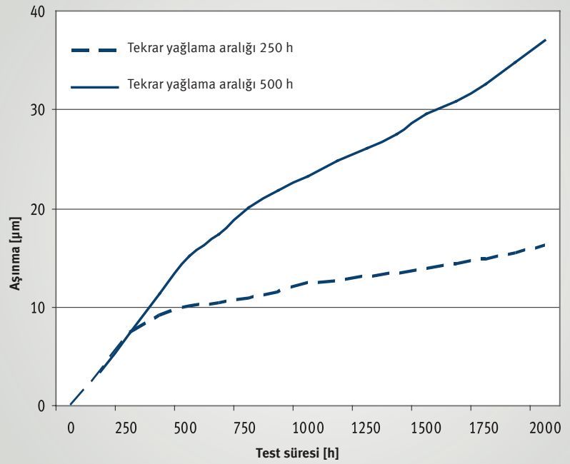
P2 kaymalı yatak aşınma eğrisi (şematik)
