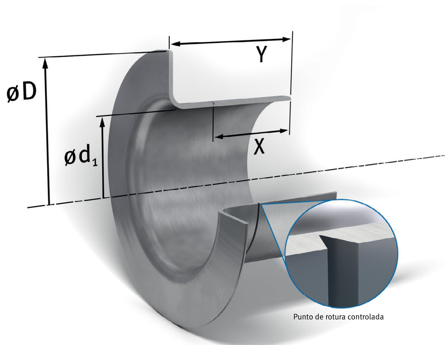
Brida de montaje separable
