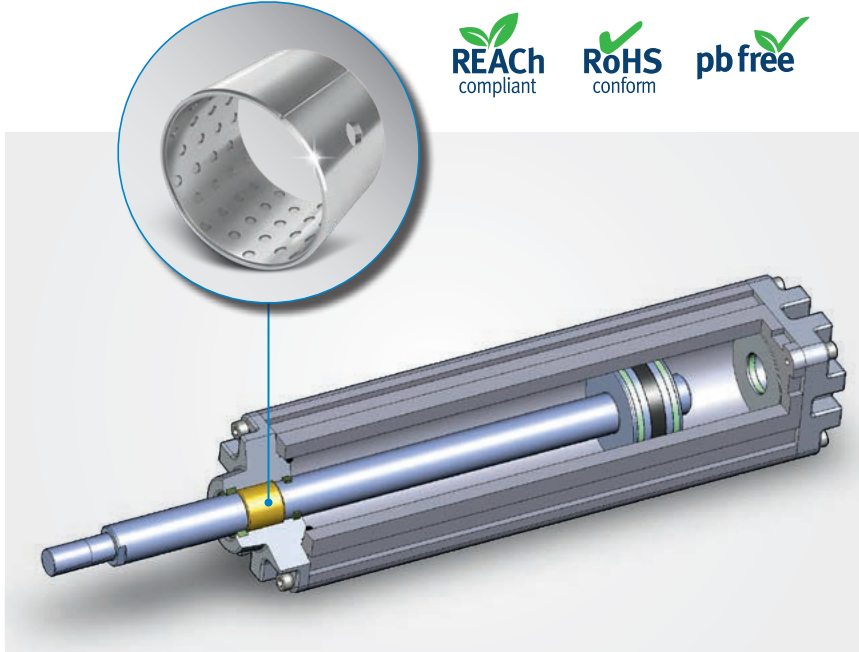
Pnömatik silindir kullanımı, KS Permaglide® P200 kaymalı yataklar aracılığıyla yataklama
