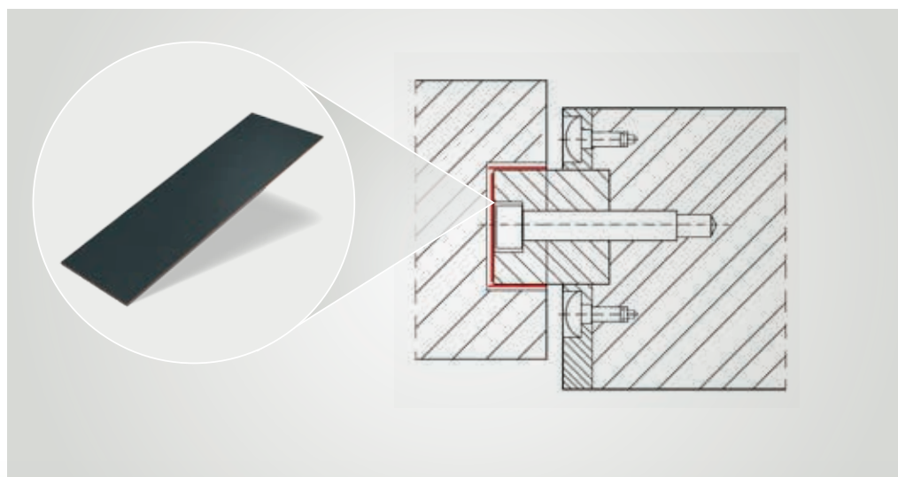
Łożyskowanie stołu przesuwного na pasmowych łożyskach ślizgowych PERMAGLIDE® typu PAS ... P11
