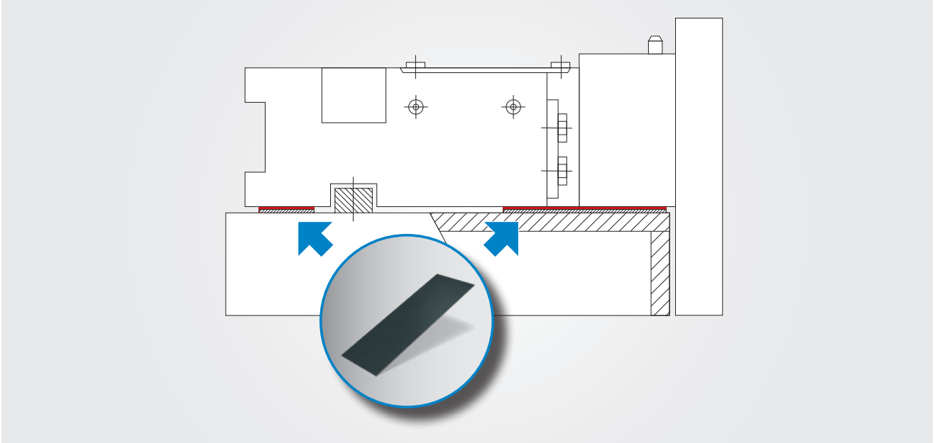
PERMAGLIDE® Yapı türü PAS ... P10 kaymalı şeritlerin olduğu bir kızak kılavuzundaki yataklamalar
