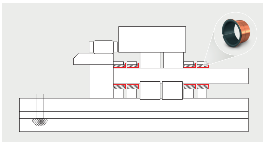
Łożyskowanie wózka łańcuchowego z tuleją z wieńcem KS PERMAGLIDE® typu PAF ... P11
