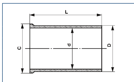
Изобр. 2: (размеры, мм)
