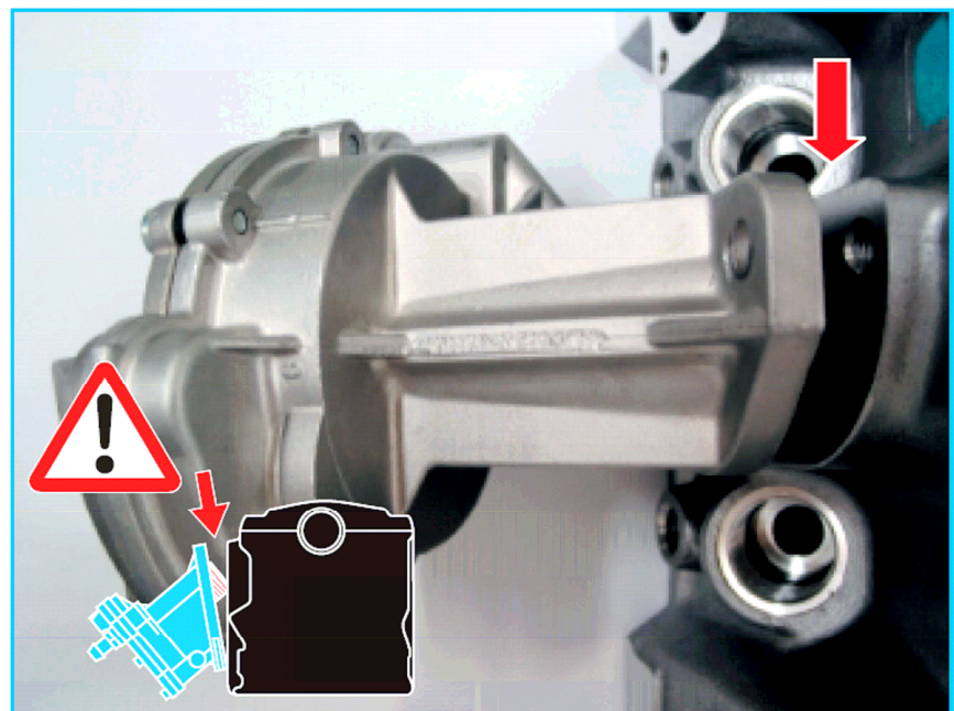
Sl. 5 U slučaju pogrešnog izbora, pravilna ugradnja nije moguća
