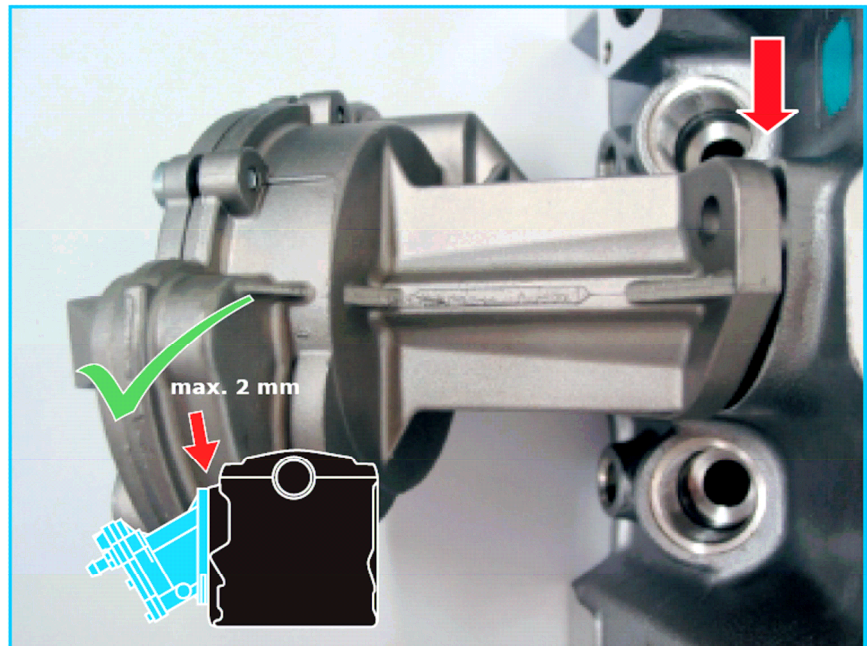
Sl. 4 Ugradnja pravilno odabrane pumpe
