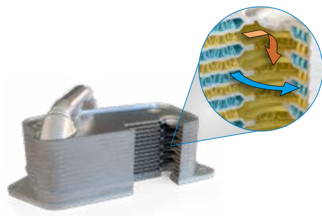
Ψυγείο λαδιού επιβατικού οχήματος
