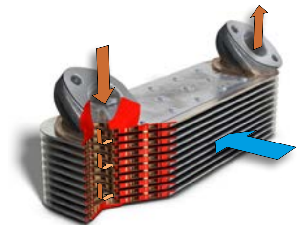
Ψυγείο λαδιού επαγγελματικού οχήματος
