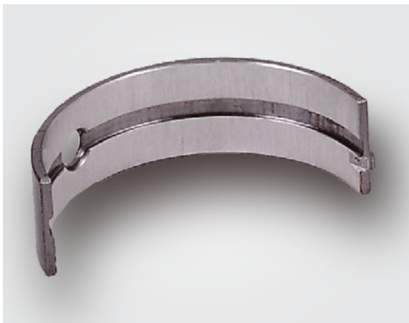
Bronzina com canal de lubrificação 72 411 6x0 - Mancal nº 2 e 4
