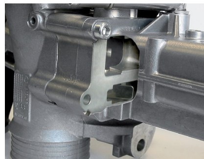
EGR 冷却器中的旁路节气门（剖面）
