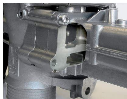
Borboleta de bypass no radiador EGR (seccionada)
