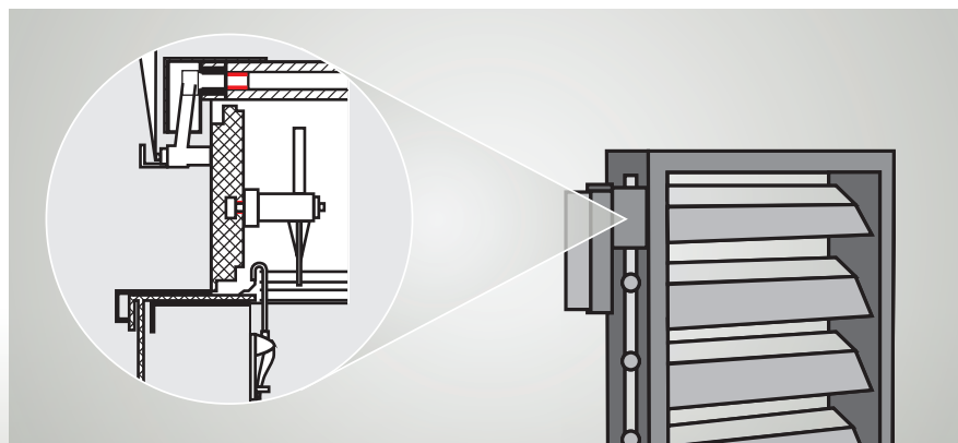
Alojamiento de las láminas mediante cojinetes PERMAGLIDE® P10
