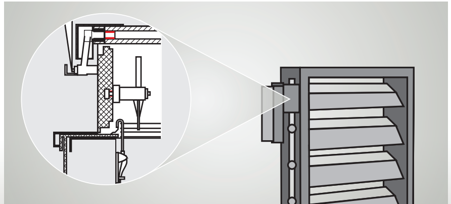
PERMAGLIDE® P10 kaymalı yataklar aracılığıyla lamel yataklaması
