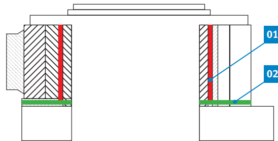
01 Tuleja łożyska ślizgowego KS Permaglide® typ PAP ... P200 02 Podkładka oporowa KS Permaglide® typ PAP ... P200
