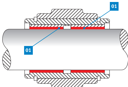
01 Tuleja łożyska ślizgowego KS Permaglide® typ PAP ... P200
