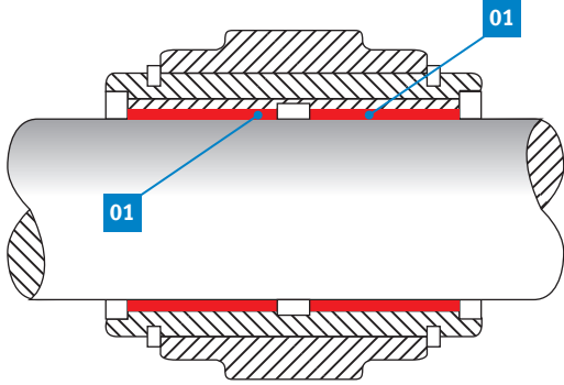
01 Permaglide® kaymalı yatak burcu Yapı türü PAP ... P200
