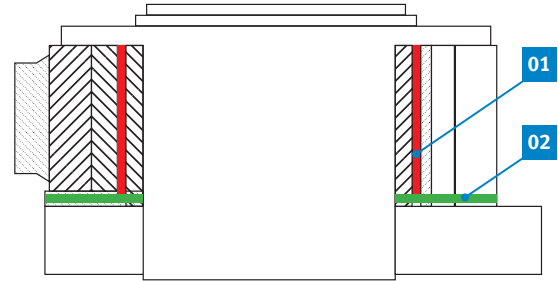
01 Permaglide® kaymalı yatak burcu Yapı türü PAP ... P200 02 Permaglide® ay yatak Yapı türü PAW ... P200
