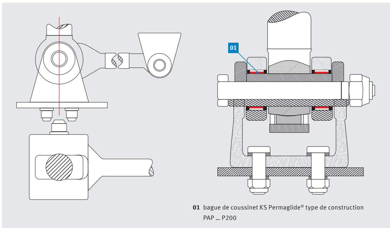
Détail articulation de basculement
