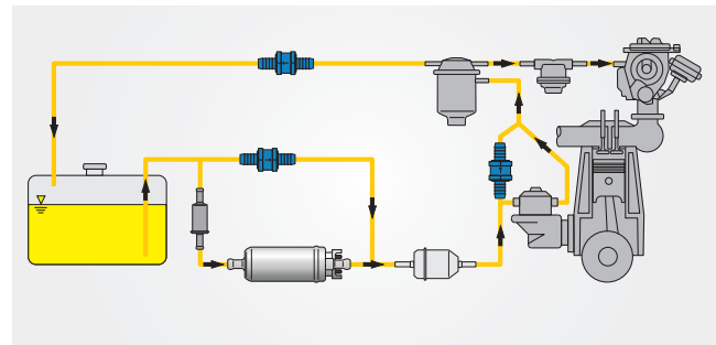
Пример применения: Карбюраторный двигатель с дополнительным подключаемым электрическим насосом
