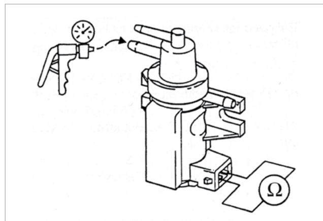
Рис. 6: Измерение электрического сопротивления клапана-преобразователя давления
