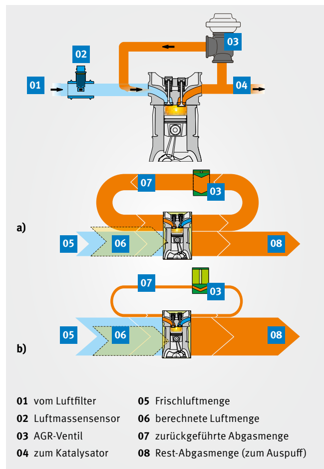
Prinzip der Abgasrückführung (AGR)
