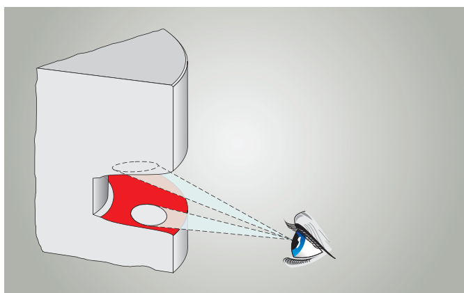
Abb.5: Sichtprüfung der Nut auf Verschleiß bei Trapezringen
