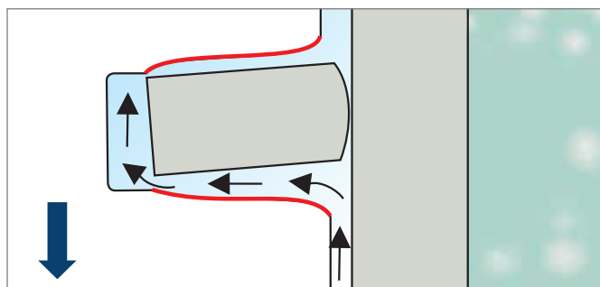
Abb. 2: Ansaugtrakt
