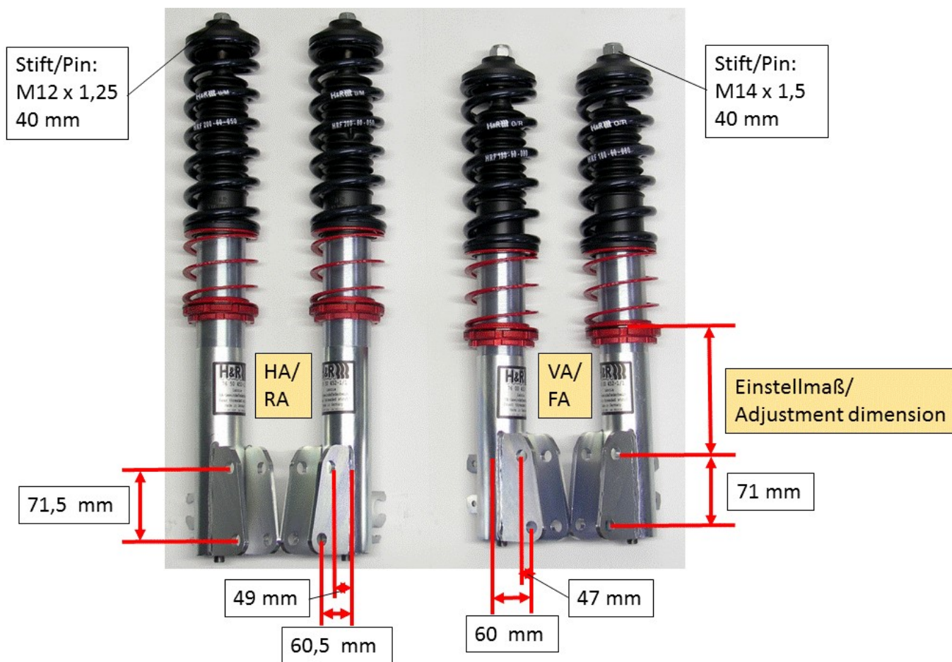
Abb. 1: Maße des H&R Fahrwerks
