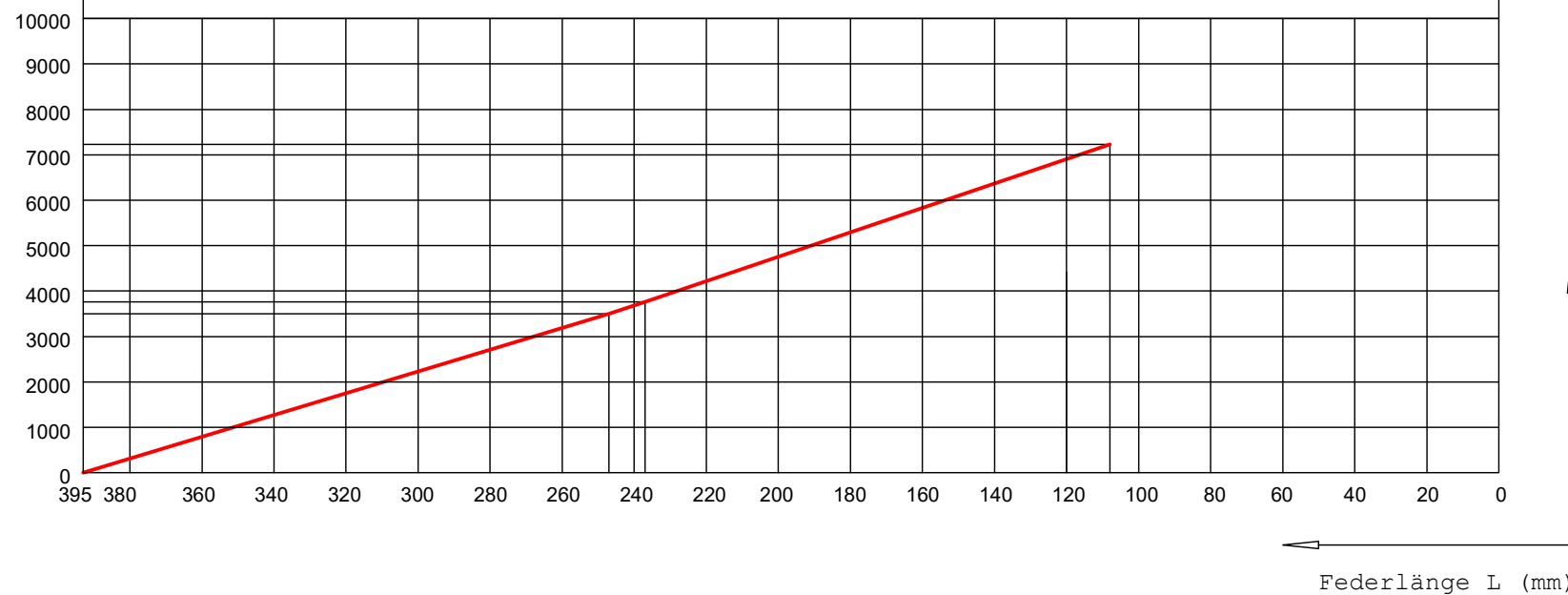
Kraft-Weg-Diagramm
