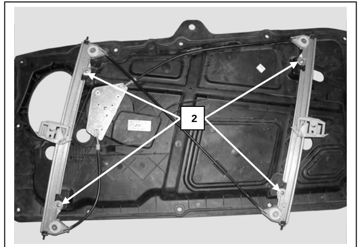
Puerta lado izquierdo, Left front door
