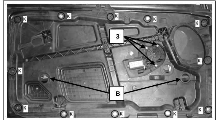
Puerta lado izquierdo, Left front door
