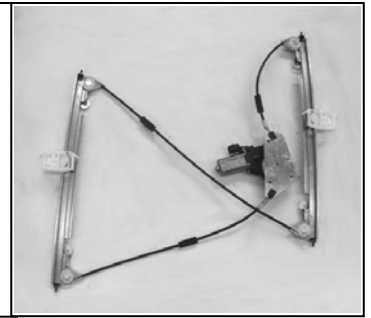
Nuestro elevallunas Our window regulator
