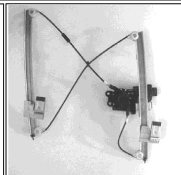
Nuestro elevallunas Our window regulator
