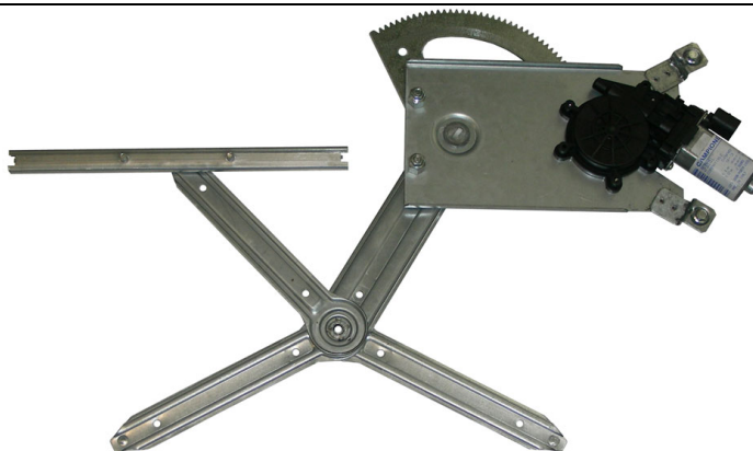
POWER WINDOW LEFT ALZACRISTALLI ELETTRICO SX
