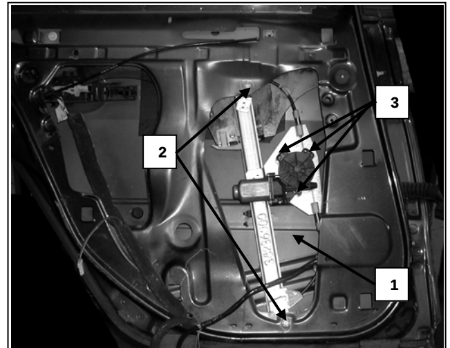
Puerta lado izquierdo, Left rear door
