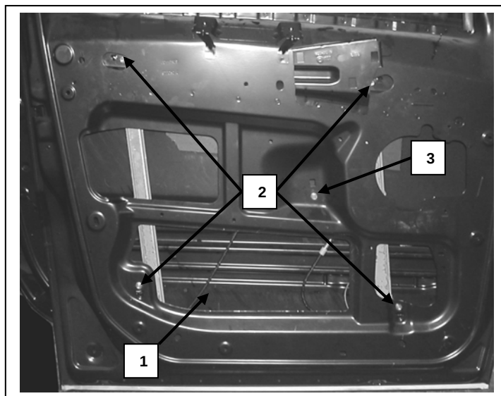
Puerta lado izquierdo, Left rear door
