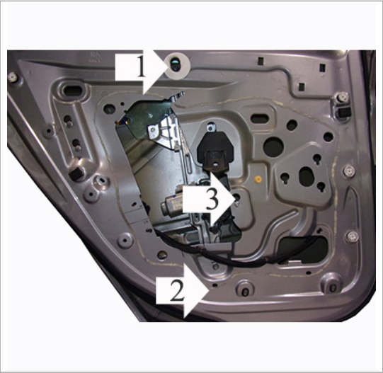
POWER WINDOW LEFT ALZCRISTALLI ELETTRICO SX
