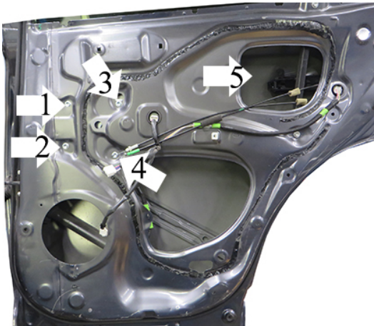
POWER WINDOW RIGHT ALZACRISTALLI ELETTRICO DX
