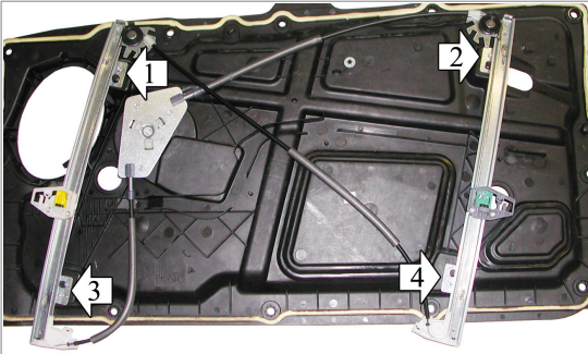
A POWER WINDOW LEFT ALZACRISTALLI ELETTRICO SX
