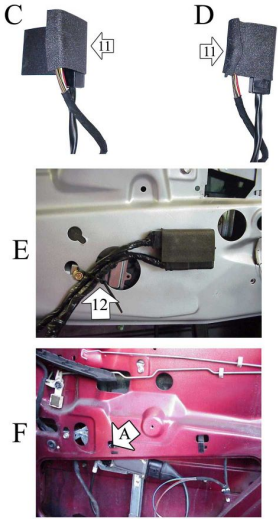
ORIGINAL POWER WINDOW RIGHT ALZACRISTALLI ELETTRICO ORIGINALE DX
