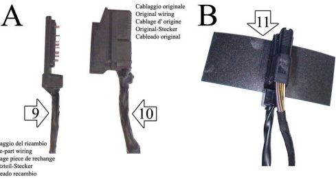
right doors - portière droite - rechte tür - puerta lado derecho - porta lato destro
