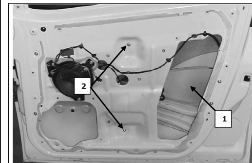
Porta lato destro, Portière avant droite, Right front door, Puerta lado derecho, Vorne rechte Tür, Porta frente dirieta, Sag on kapı, πόρτα εμπρός δεξιά
