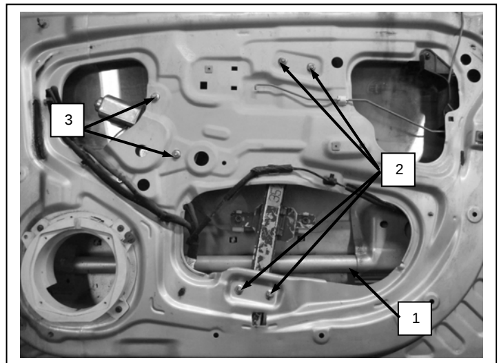
Porta lato destro, Portière avant droite, Right front door, Puerta lado derecho, Vorne rechte Tür, Porta frente dirietta, Sag on kapi, πόρτα εμπρόςθια δεξιά
