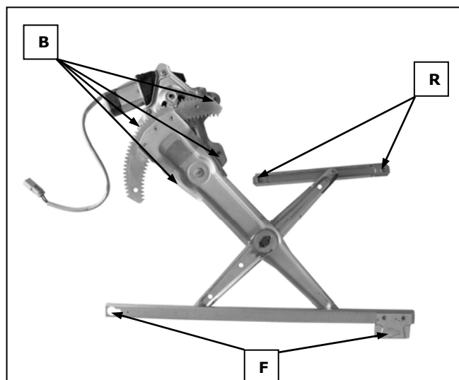
Nostro alzacrystallo - our window regulator - notre lève-vitre - unser Fensterheber - nuestro elevalunas - nosso levantador de vidro - bizim cam acacagi - Γρύλος δικός μας
