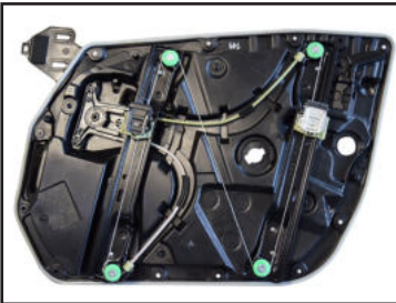
Alzacristallo originale - oem window regulator - lève-vitre original - Fensterheber von oem - elevallunas original - levantator de vidro original - orijinal cam acacagi - Γρύλος γνήσιος
