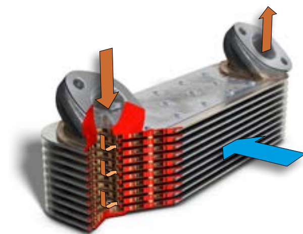
商用车油冷器
