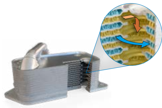
客车用油冷器
