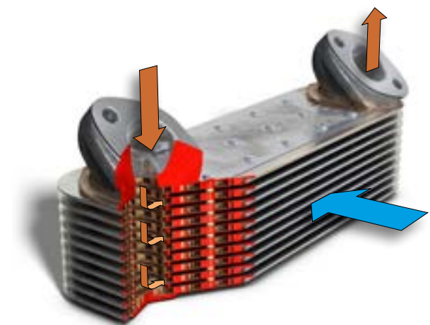
Refrigerador de aceite para vehículos comerciales
