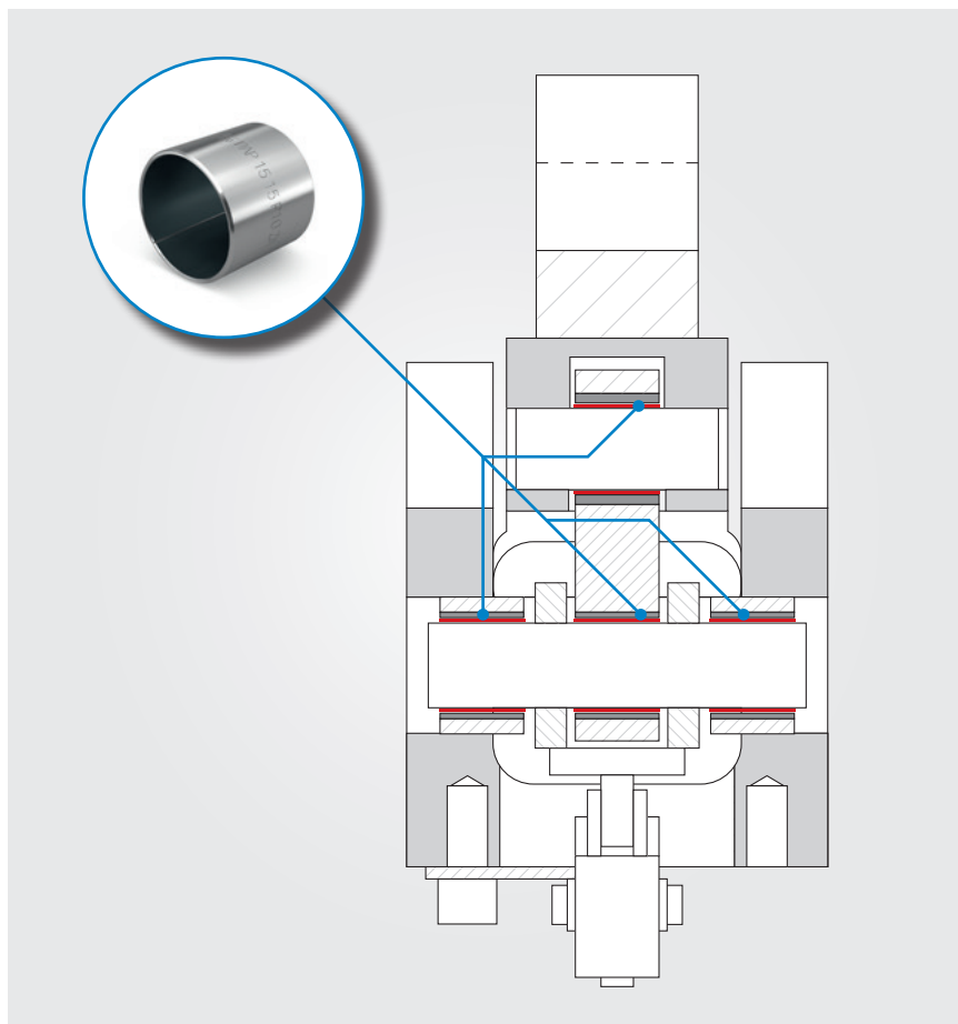
łożyskowanie sworzni w zaciskach kolanowych tulejami łożysk ślizgowych PERMAGLIDE® typu PAP ... P10
