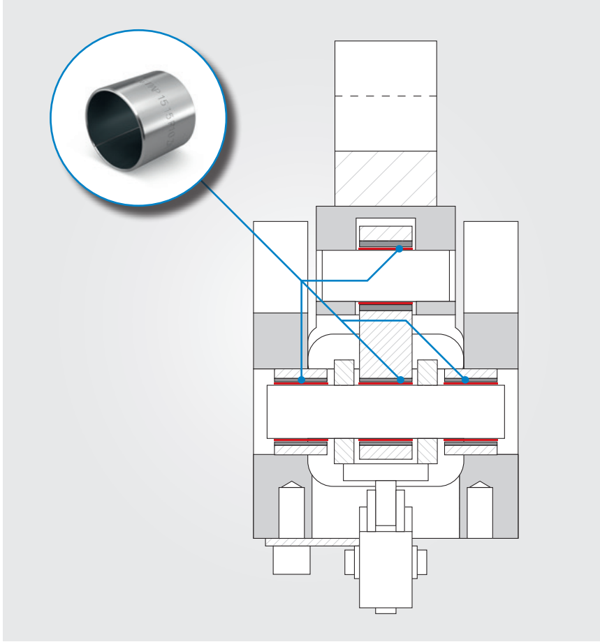
PERMAGLIDE® Yapı türü PAS ... P10 kaymalı şeritlerin olduğu bir diz manivelası ile sıkıştırıcıdaki pim yatakları
