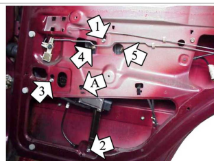
POWER WINDOW RIGHT ALZACRISTALLI ELETTRICO DX
