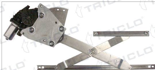
POWER WINDOW RIGHT ALZACRISTALLI ELETTRICO DX
