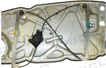
POWER WINDOW LEFT ALZACRISTALLI ELETTRICO SX
