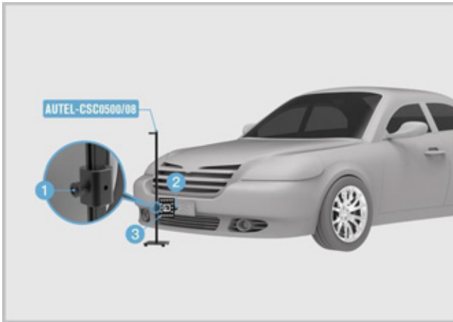
Abbildung 6-68 Einstellen der Distanzmessscheibe
