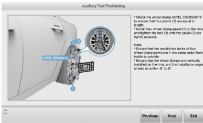
Bild 5-45 Positionierung des Hilfswerkzeugs 4
