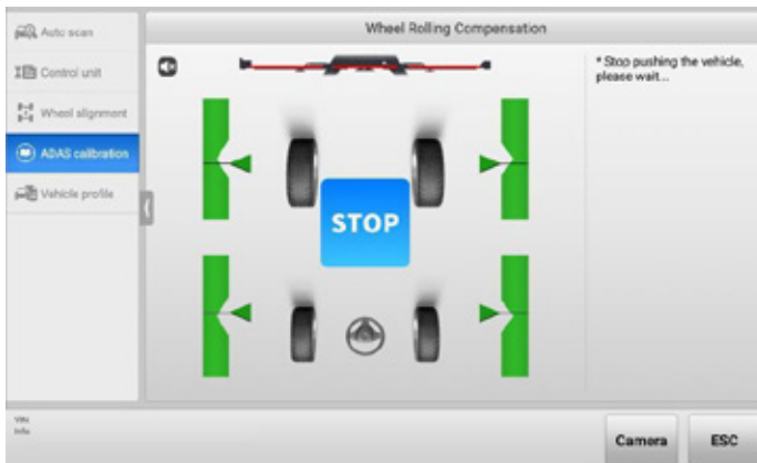
Bild 6-96 Radrollkompensation 4
