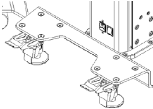
Abbildung 2-5 Zwei Fußbremsen
