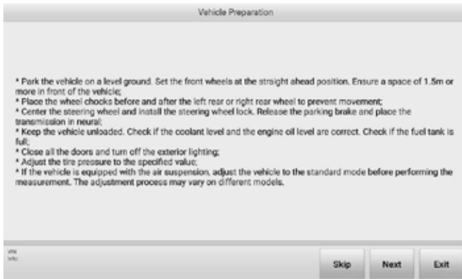
Abbildung 5-41 Fahrzeugvorbereitung
