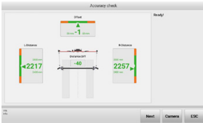
Abbildung 5-37 Bildschirm "Genauigkeitsprüfung" (Kalibrierungsleiste verwenden) 3
