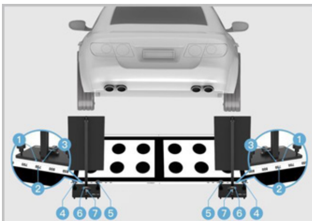
Abbildung 6-54 Kalibrierung der Kamera Rückseite 2
