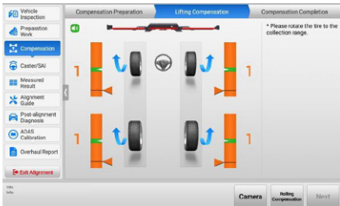
Bild 4-45 Start des Hebeausgleichs 4 (Felgenklemme verwenden)
