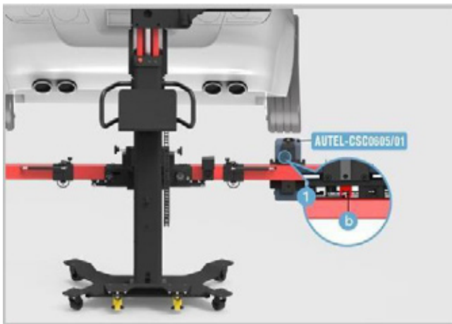
Bild 6-49 Verschieben der Radarkalibrierungsbox (rechts)
