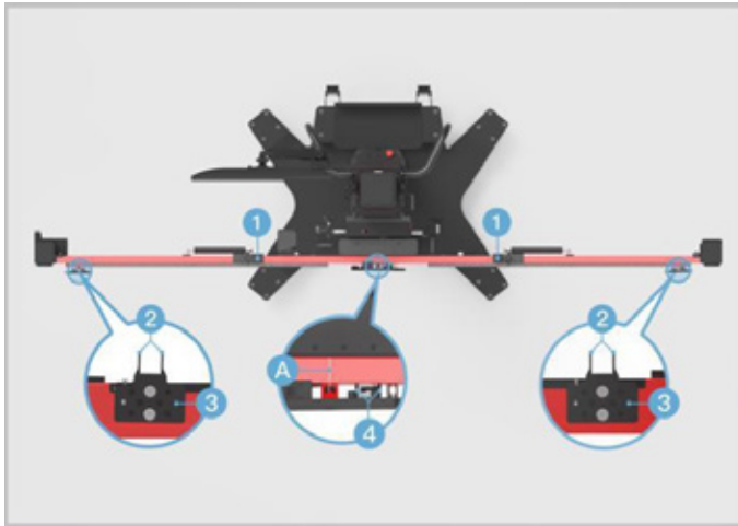
Abbildung 6-36 Positionieren der Schiebeplatte
