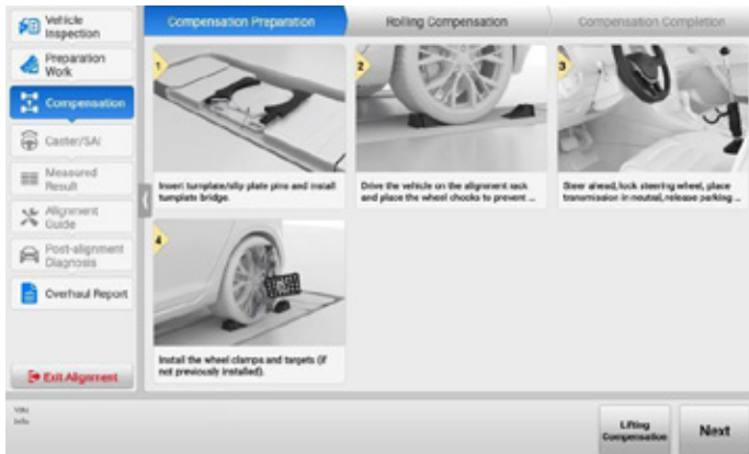
Bild 4-35 Vorbereitungen für den Rollausgleich (Felgenklemme verwenden)
