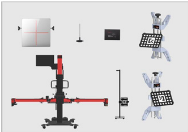
Abbildung 6-1 Erforderliche Kalibrierwerkzeuge
