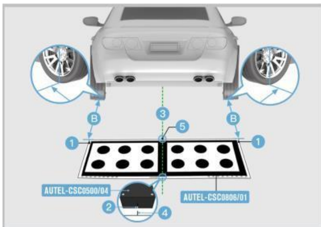
Abbildung 6-53 Kalibrierung der Kamera Rückseite 1
