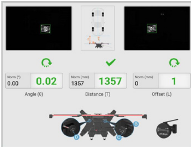
Abbildung 6-7 Einstellen des Kalibrierungsrahmens
