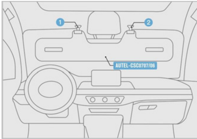
Bild 6-60 HUD-Kalibrierungsplatine platzieren
