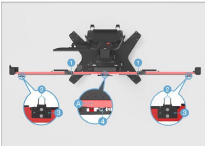
Bild 6-64 Schiebepatte positionieren
