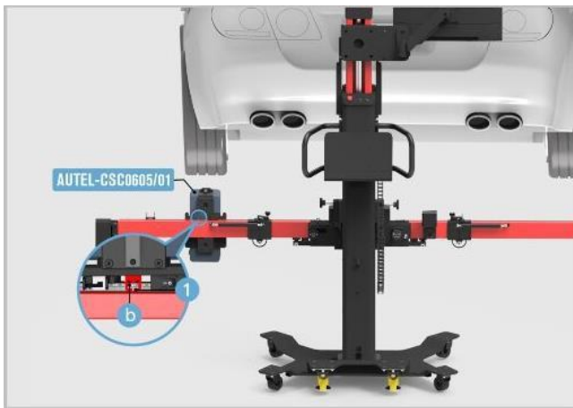
Abbildung 6-33 Verschieben der Radarkalibrierungsbox (links)
