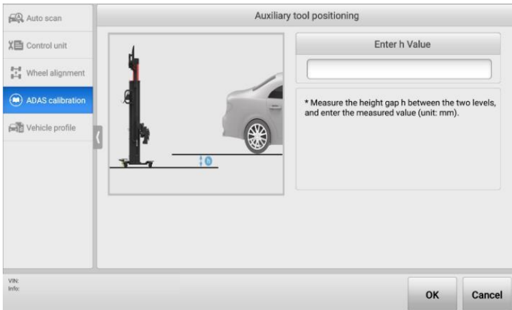
Abbildung 6-23 Messwert h
