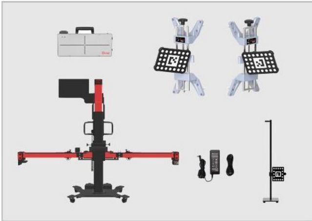
Abbildung 6-63 Erforderliche Kalibrierwerkzeuge
