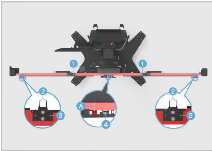
Bild 6-77 Schiebepatte positionieren
