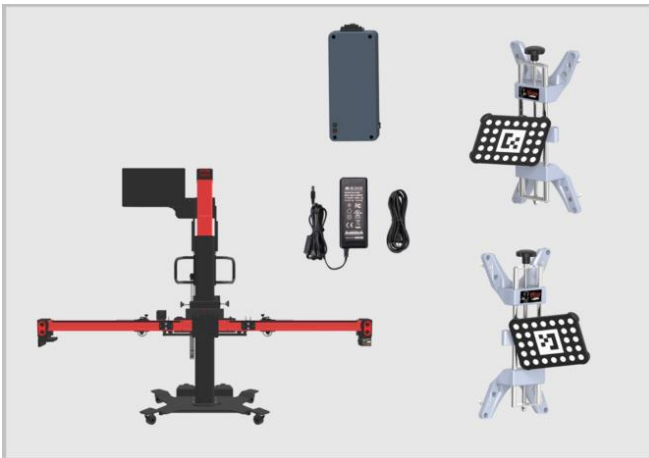
Abbildung 6-24 Erforderliche Kalibrierwerkzeuge (bei Auswahl von A oder B)
