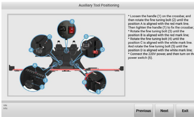
Bild 5-43 Positionierung des Hilfswerkzeugs 2
