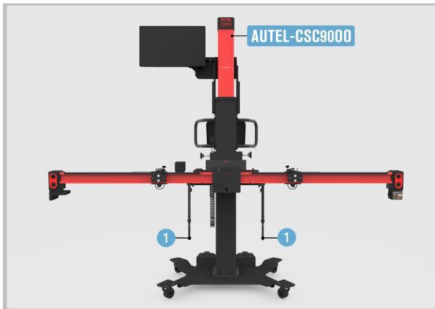
Bild 6-84 Halterung für Zielplatte erweitern
