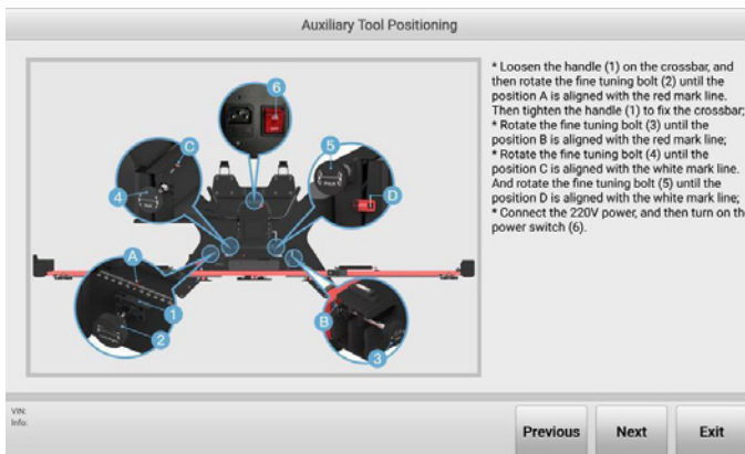
Bild 5-52 Positionierung des Hilfswerkzeugs 2
