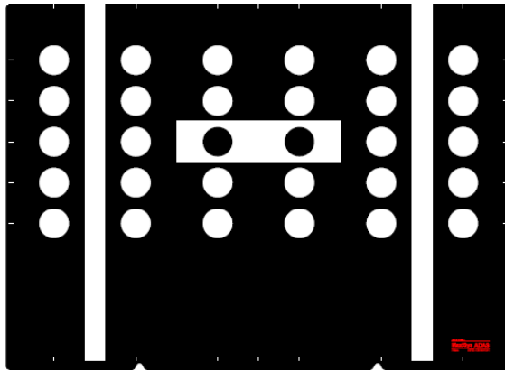
Abbildung 3-47 Musterkarte AUTEL-CSC0601/01
