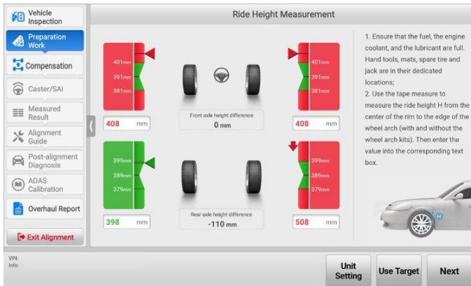
Abbildung 4-30 Messen der Fahrzeughöhe mit Maßband 1
