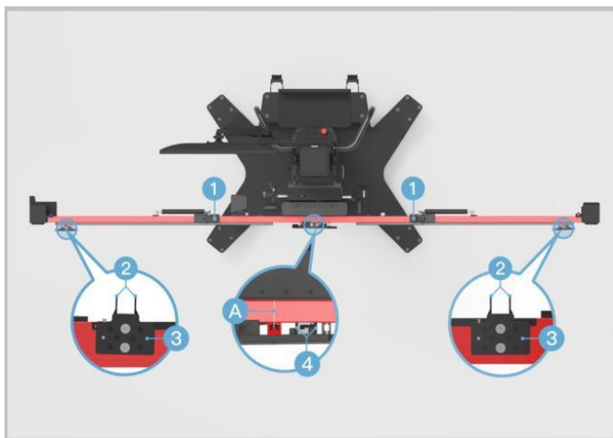
Bild 6-77 Schiebeplatte positionieren
