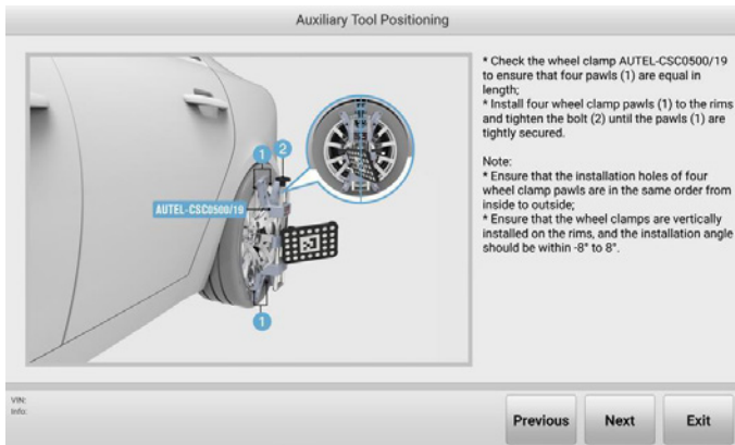
Bild 5-54 Positionierung des Hilfswerkzeugs 4
