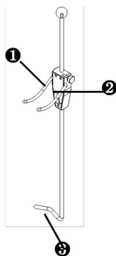
Abbildung 3-3 Bremspedal-Drücker AUTEL-CSC0500/26
