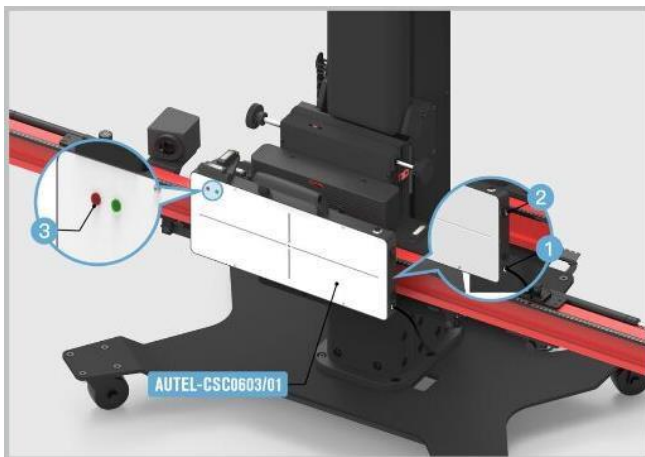
Abbildung 6-71 Strom anschließen
