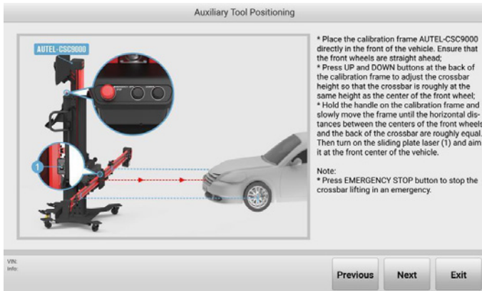
Bild 5-53 Positionierung des Hilfswerkzeugs 3
