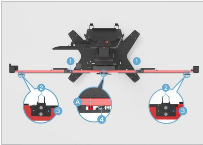
Bild 6-89 Schiebeplatte positionieren
